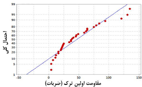
شکل ۱۷- نمودار احتمال مقاومت اولین ترک NC (خشک)
