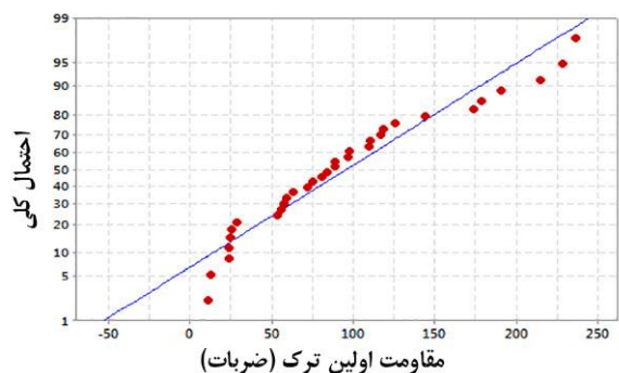
شکل ۱۵- نمودار احتمال مقاومت اولین ترک HST (مرطوب)
