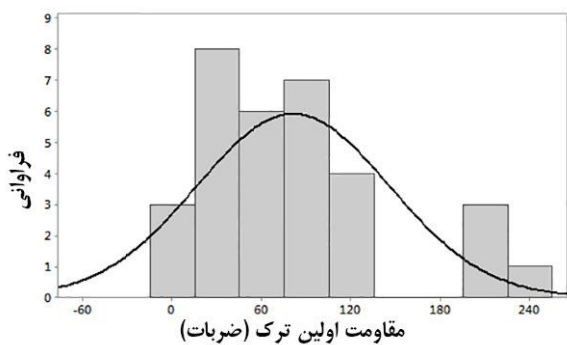
شکل ۲۲- نمودار هیستوگرام مقاومت اولین ترک SFC5 (خشک)
