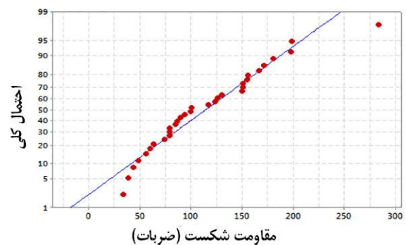
شکل ۳۱- نمودار احتمال مقاومت شکست SFC2 (مرطوب)
