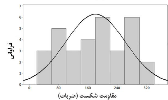
شکل ۳۲- نمودار هیستوگرام مقاومت شکست SFC5 (مرطوب)
