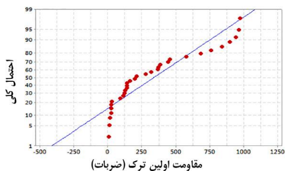
شکل ۷- نمودار احتمال مقاومت اولین ترک SFH3 (مرطوب)
