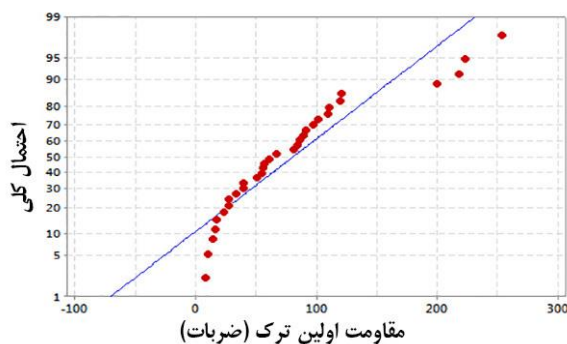
شکل ۲۳- نمودار احتمال مقاومت اولین ترک SFC5 (خشک)
