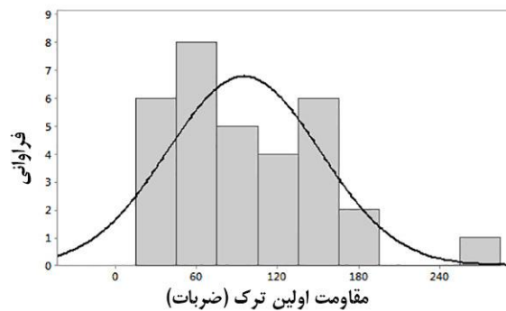
شکل ۸- نمودار هیستوگرام مقاومت اولین ترک SFC2 (مرطوب)
