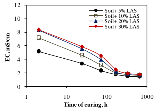
شکل ۳- تغییرات هدایت الکتریکی (EC) خاک در حضور آهک، سرباره کنورتور و زمان‌های متفاوت عمل‌آوری
