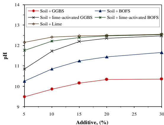
شکل ۴- تغییرات pH نمونه‌ها بر اثر اندرکنش خاک با مواد اصلاح‌کننده مورد مطالعه
