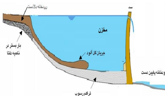
شکل ۱- شکل شماتیک اجزای یک جریان گل‌آلود
