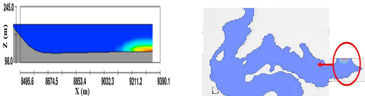
شکل ۱۰- زبانه جریان غلیظ ورودی به ایستگاه F در بالادست مخزن سد دز
