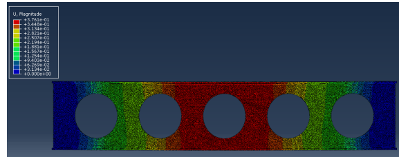
شکل ۶- تغییر شکل تیر لانه زنبوری با سوراخ‌های دایره‌ای شکل تحت اثر بار ۸/۵
