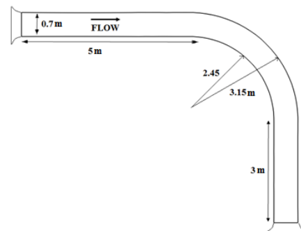
شکل ۲- شکل شماتیک فلوم آزمایشگاهی
