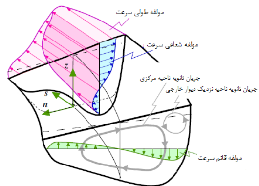
شکل ۱- الگوی جریان شکل گرفته در کانال قوسی شکل (نشریه ۵۱۶، ۱۳۸۸)
