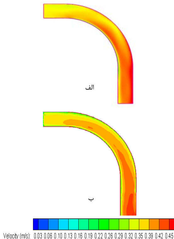
شکل ۴- الگوی سرعت پیش‌بینی شده توسط: الف) مدل CCHE2D، ب) مدل SRH-2D
