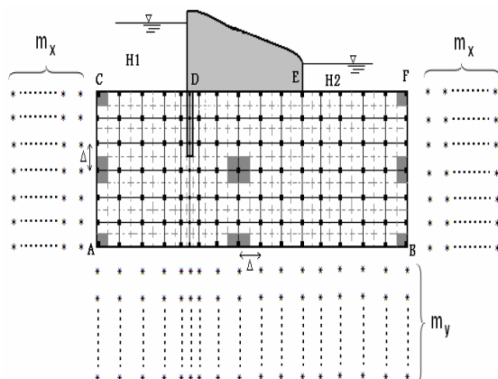
شکل ۱- نحوه شبکه بندی محیط زیر سد بتنی نمونه
