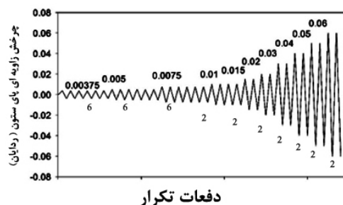
شکل 12- نمودار جابه‌جایی چرخه‌ای اعمال شده به سازه به روش SAC
