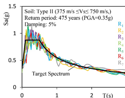
شکل 14- مقایسه طیف شتاب‌نگاشت‌های مصنوعی با طیف طراح ساخت
