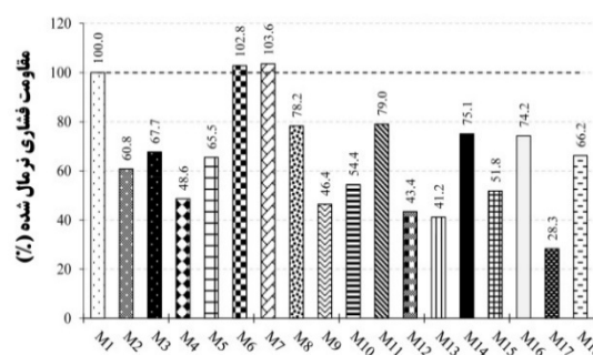
شکل 3- مقاومت فشاری نرمال شده نمونه‌های ملات
