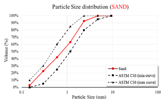
شکل 1- منحنی دانه بندی ماسه
