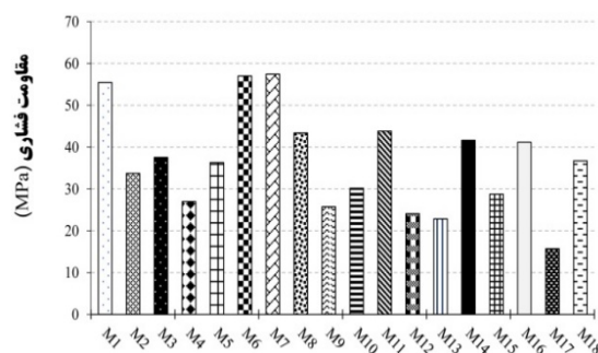
شکل 2- مقاومت فشاری نمونه‌های ملات
