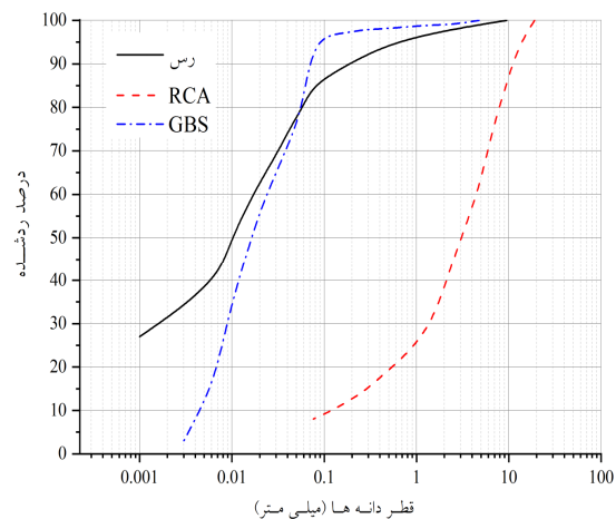
شکل 1- منحنی دانه‌بندی مصالح استفاده شده در تحقیق حاضر
