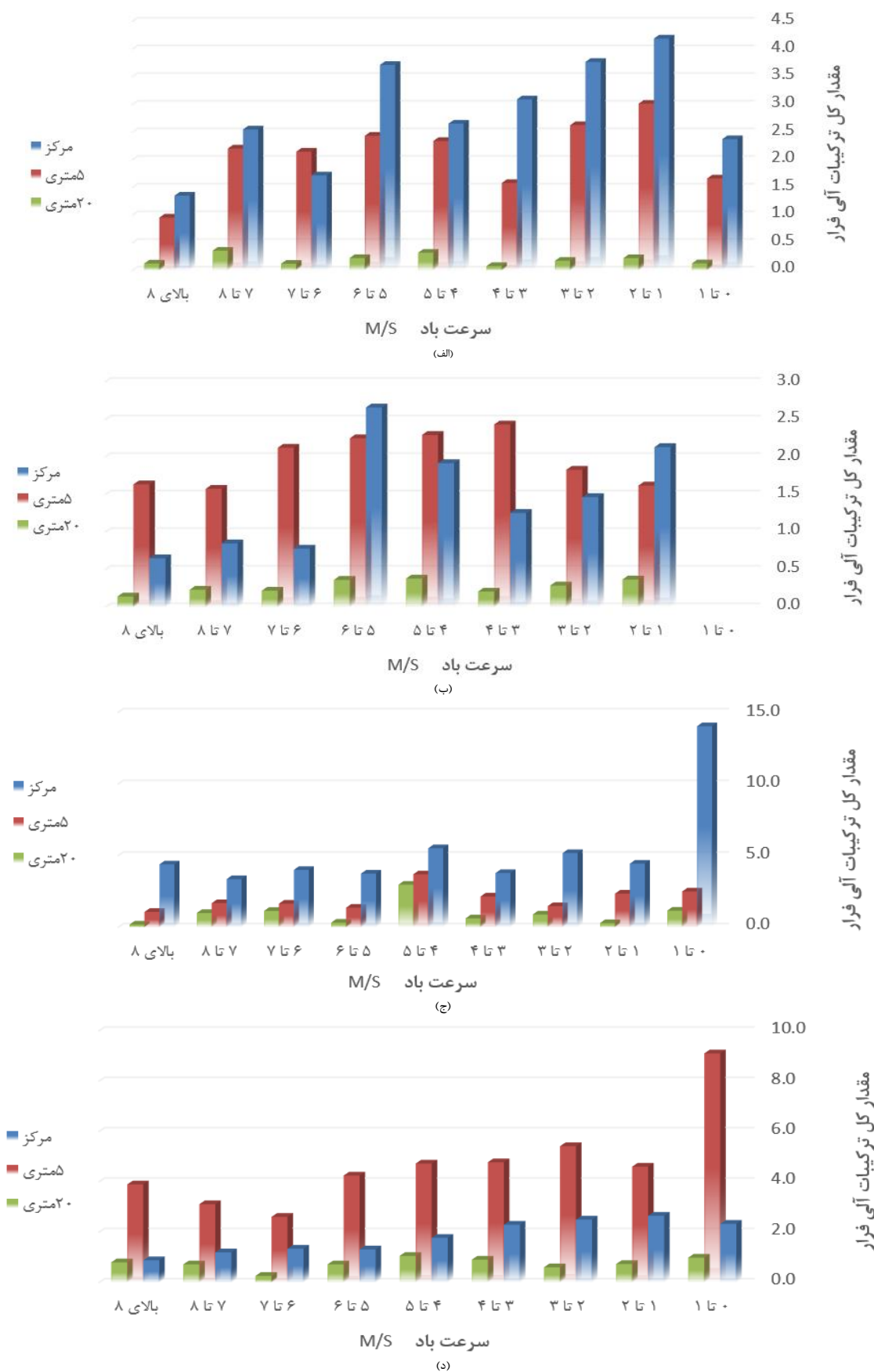
شکل ۷- تغییرات غلظت ترکیبات آلی فرار با سرعت باد در ۴ جایگاه منتخب برحسب ppm: (الف) آذربایجان، (ب) تعاونی ۱۰۶، (ج) تعاونی ۴۵، (د) مجید
