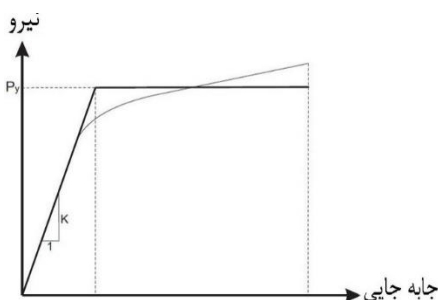
شکل ۸- منحنی ساده شده نیرو تغییر مکان
