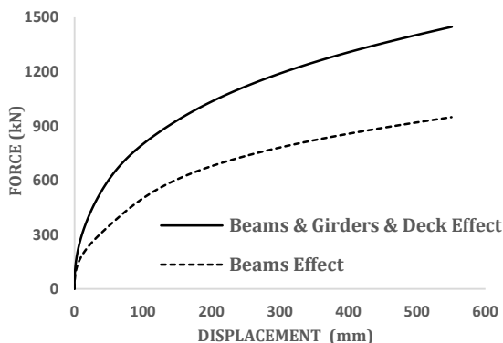
شکل ۱۱- نمودارهای نیرو- جابه‌جایی برای حالت ۱۵ در محل حذف ستون A و B
