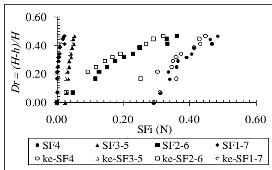
شکل ۸- مقایسه نیروی برشی المان مرزی در کانال مرکب منشوری با سیلاب‌دشت‌هایی به عرض: الف) ۱۰۰، ب) ۲۰۰، ج) ۳۰۰، د) ۴۰۰ میلی‌متر
