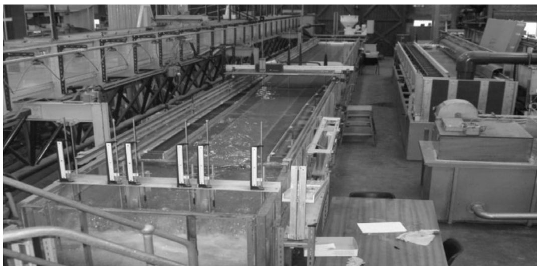
شکل ۱- تصویر کانال آزمایشگاهی
