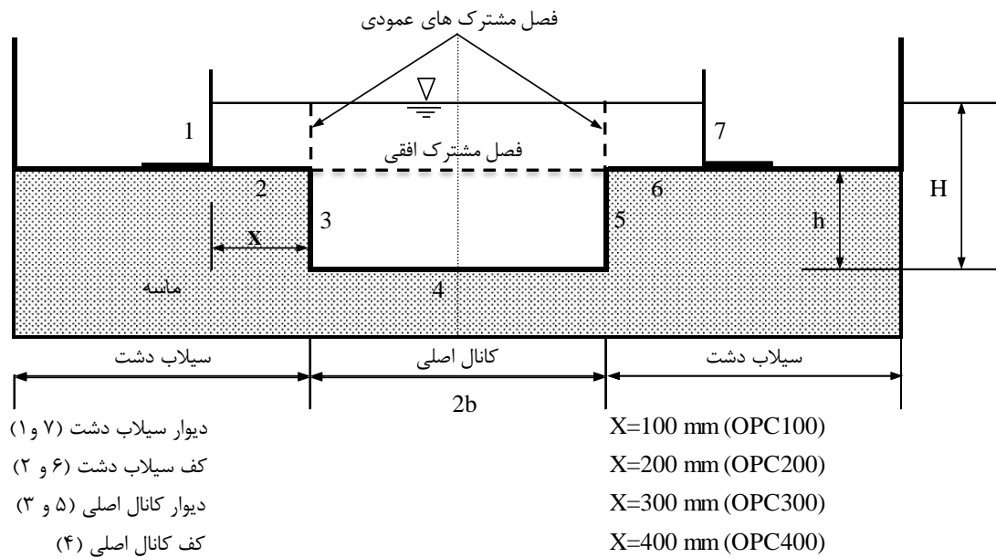
شکل ۲- مقطع عرضی کانال تحقیقاتی
