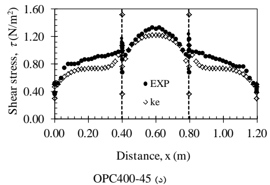
شکل ۷- توزیع تنش برشی دیواره برای دبی ۴۵ لیتر بر ثانیه در سیلاب‌دشت‌هایی به عرض: الف) ۱۰۰، ب) ۲۰۰، ج) ۳۰۰، د) ۴۰۰ میلی‌متر
